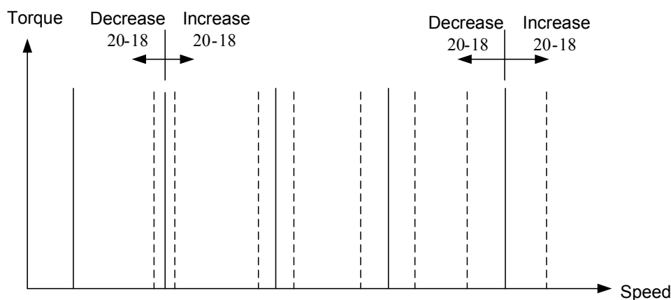
圖 4.3.116 20-18 對於轉矩-速度曲線的影響
