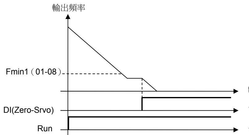
圖 4.3.129 零伺服定位示意圖
