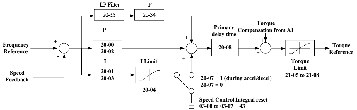
圖 4.3.109 速度控制架構(SV 模式及 PMSV 模式)
