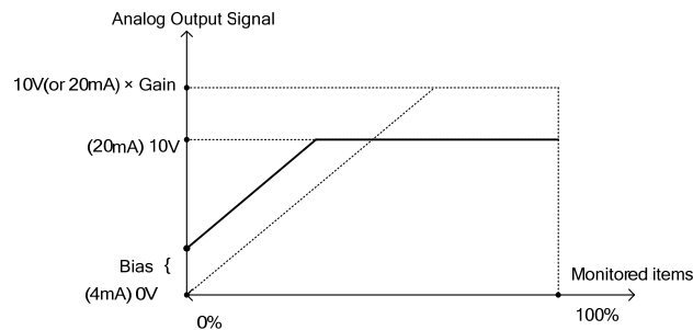
圖4.3.51 類比輸出準位調整
