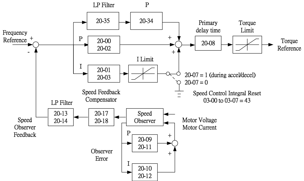
圖 4.3.108 速度控制架構(SLV 模式)
