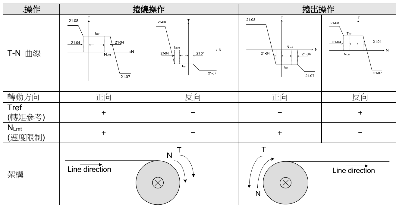
圖 4.3.126 捲繞和捲出操作
