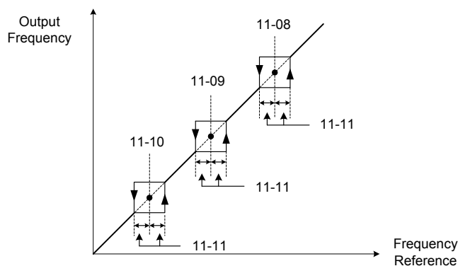
圖4.3.86 跳躍頻率操作
