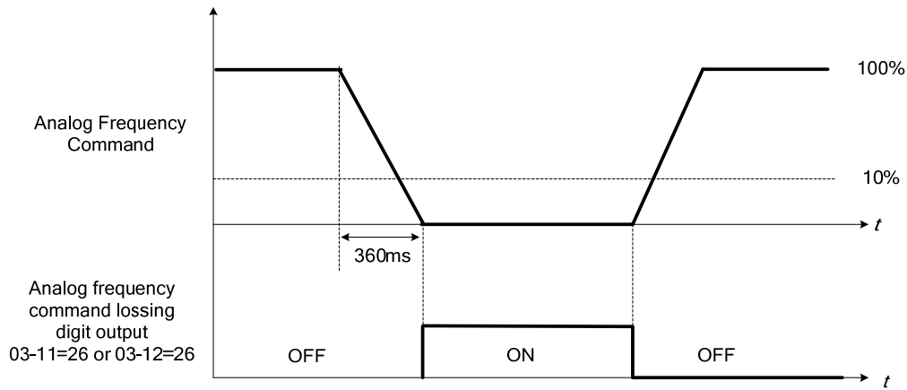
圖 4.3.93 頻率參考遺失操作
