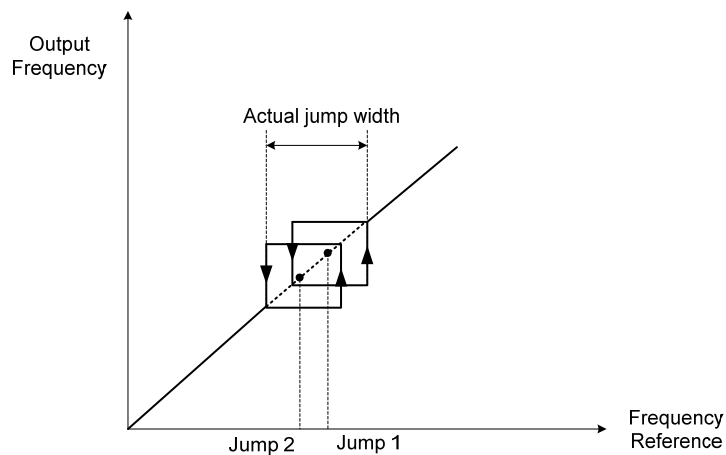
圖4.3.87 跳躍頻率重疊
