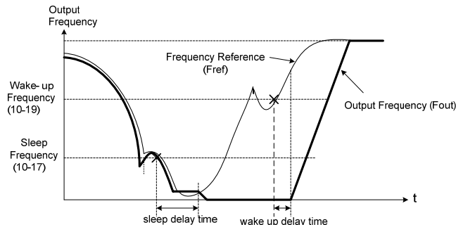
(b) PID 休眠/喚醒之時序圖
