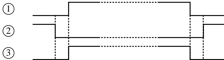
電磁接觸器動作時序圖
