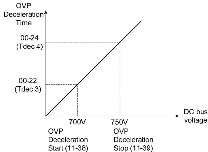
圖 4.3.92 OVP減速時間
