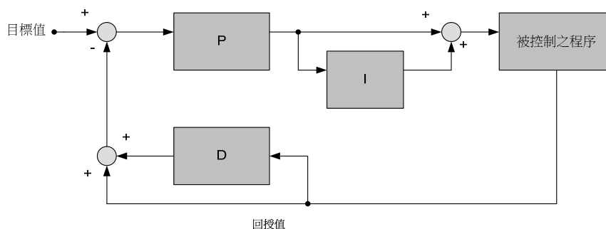
圖 4.3.78 回授微分值 PID 控制
