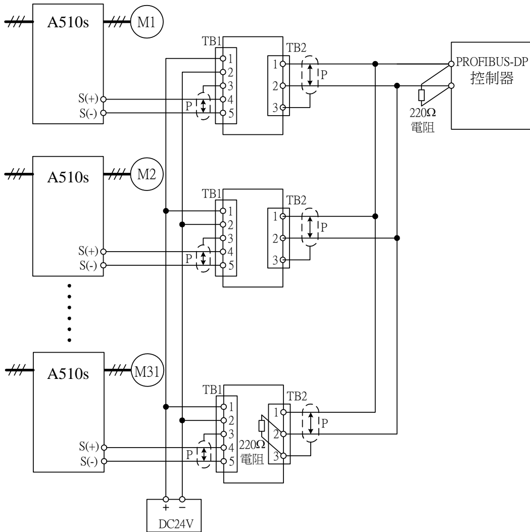
PROFIBUS 通訊協定之配線圖
