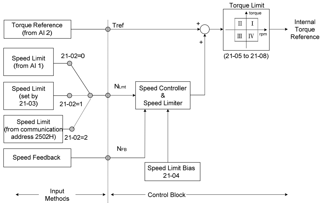
圖 4.3.121 轉矩控制方塊圖
