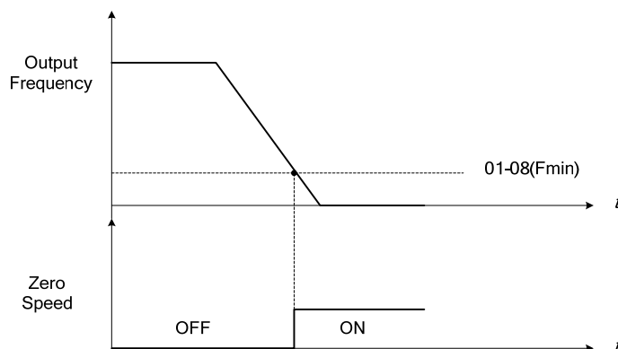
圖4.3.26 零速度操作
