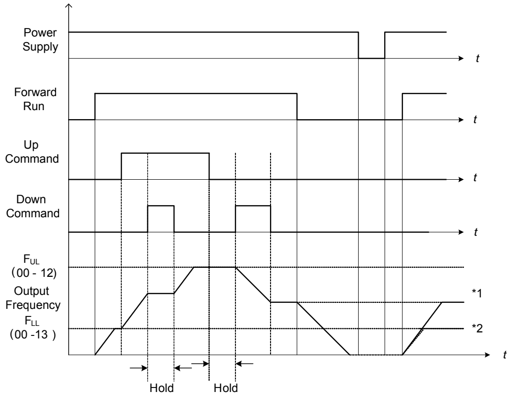
圖 4.3.20 Up / Down指令時序圖
