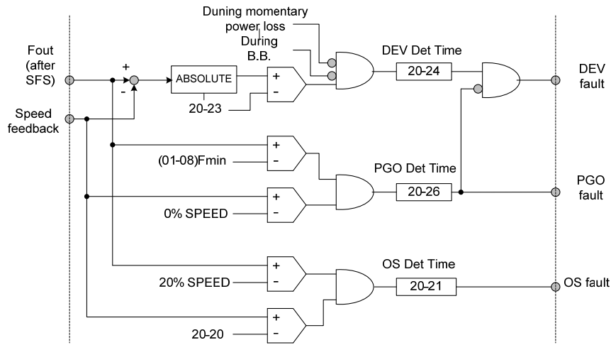
圖 4.3.117 PG 回授故障偵測方塊圖
