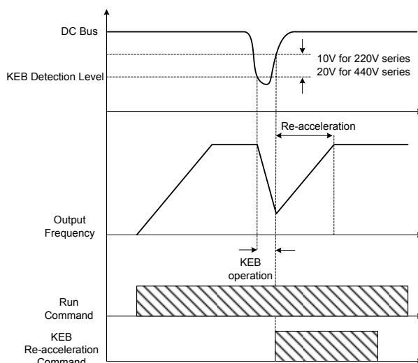
圖 4.3.95 KEB 操作
