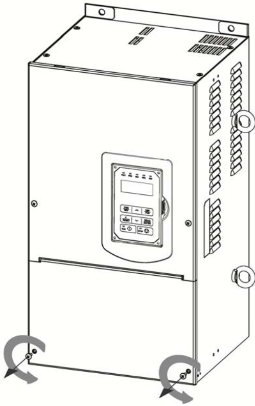
步驟一：鬆開螺絲
