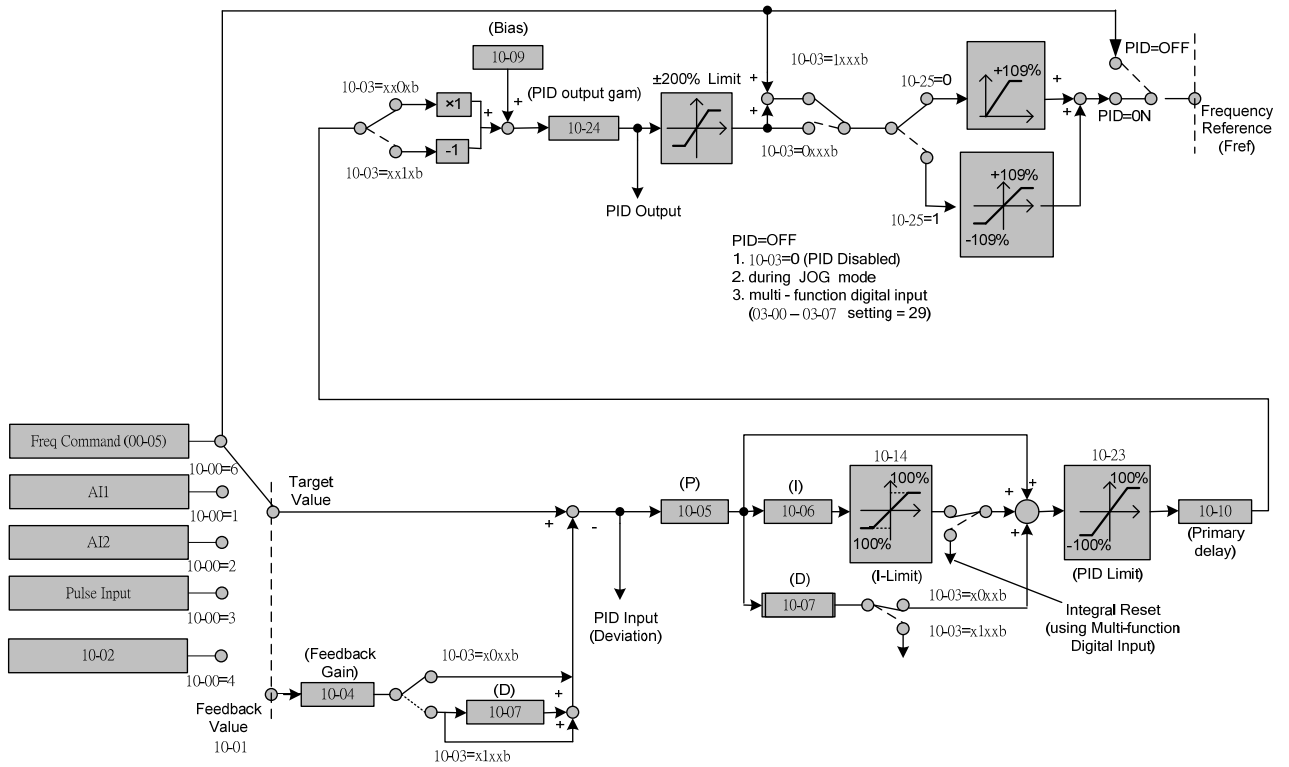
圖 4.3.81 PID 控制方塊圖
