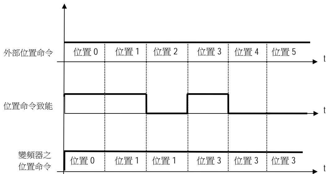
圖 4.3.131 位置致能示意圖
