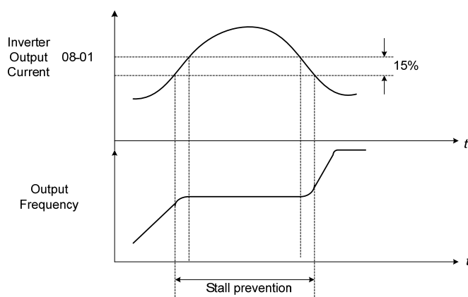
圖. 4.3.67 加速期間失速防止
