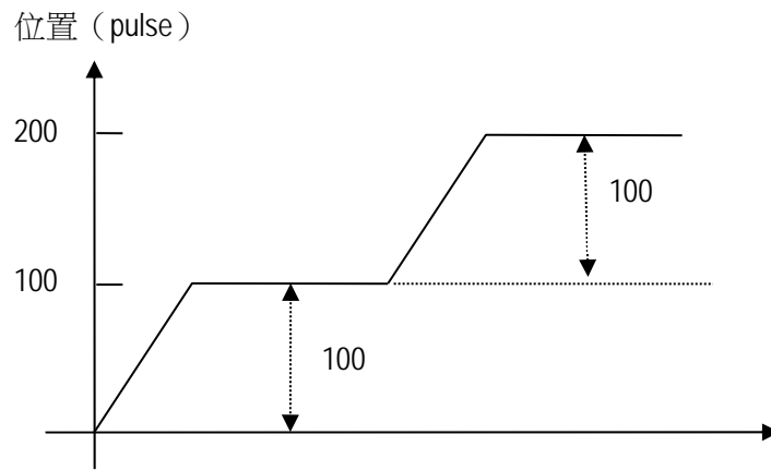
圖 4.3.132 絕對型示意圖
