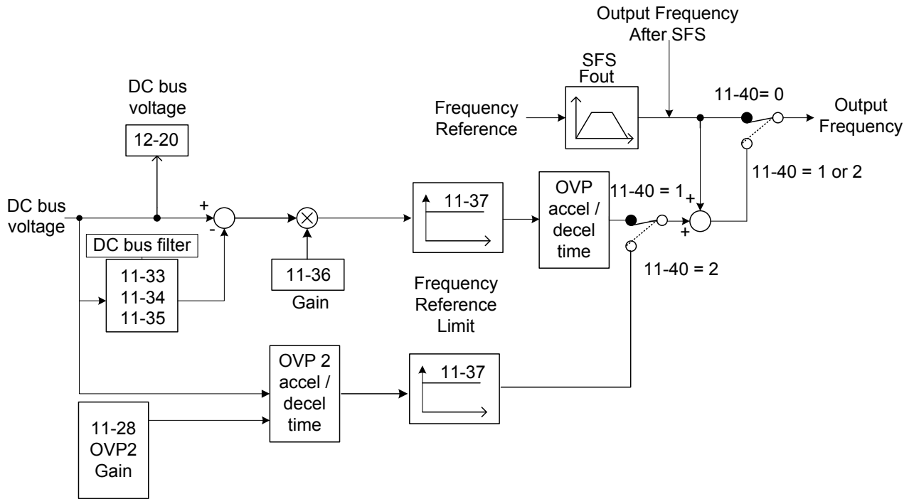
圖 4.3.91 OVP操作
