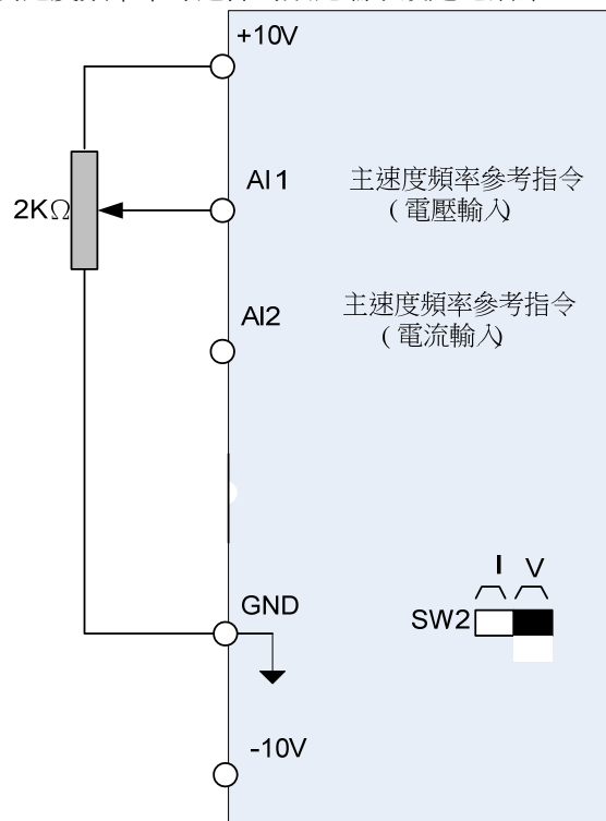
圖 4.3.4 主速度頻率參考指令之類比輸入
