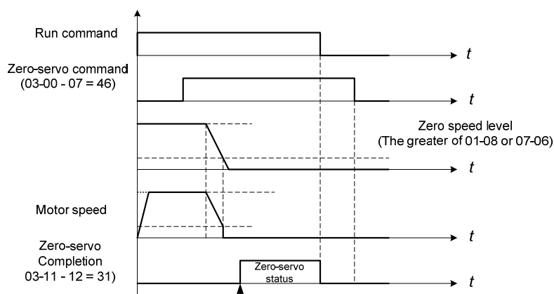
圖 4.3.96 零伺服操作
