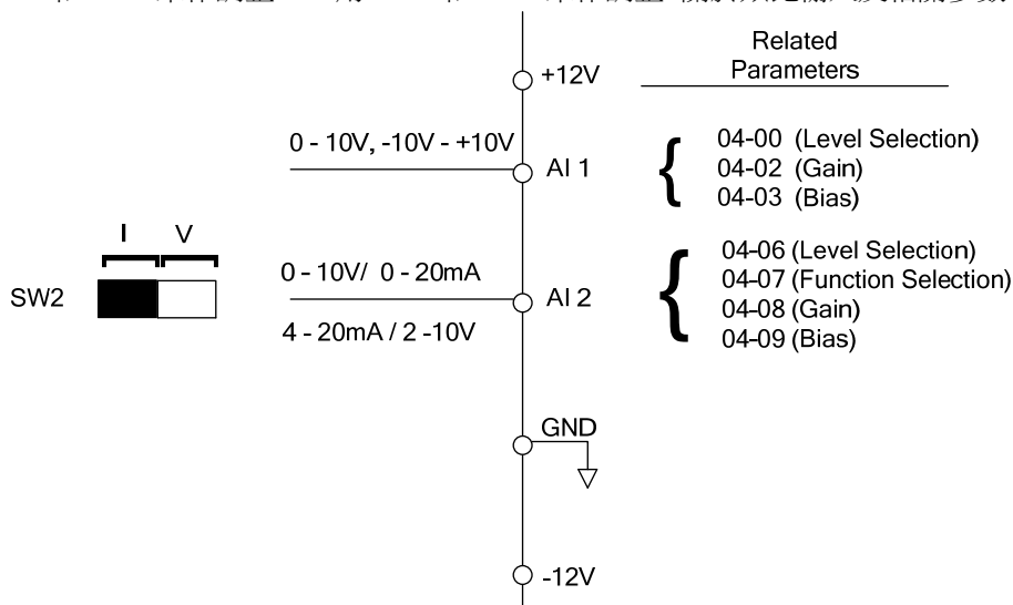
圖4.3.35 類比輸入及相關參數
