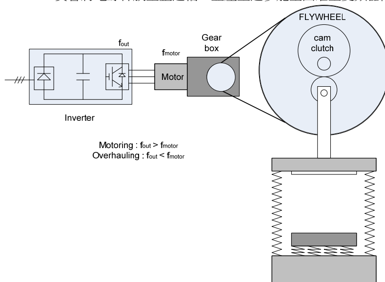
圖 4.3.90 沖壓操作
