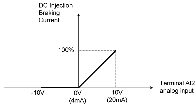
圖4.3.44 直流剎車電流調整
