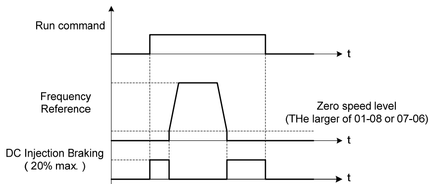
圖 4.3.97 零速度剎車操作
