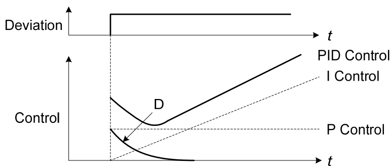
圖 4.3.77 PID 控制操作
