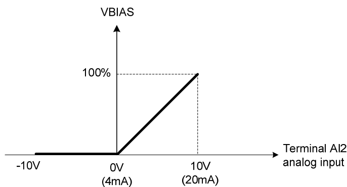
圖4.3.42 偏壓調整
