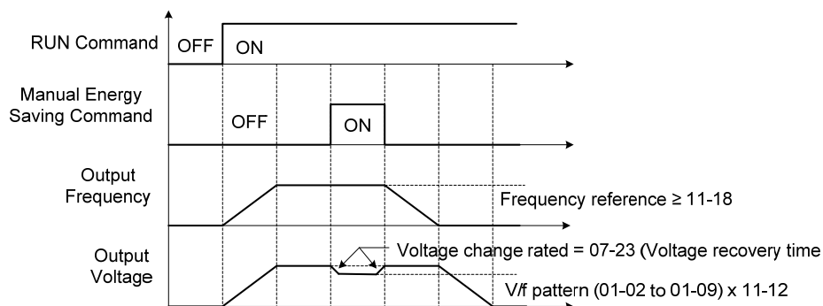
圖 4.3.88 手動節省能源操作
