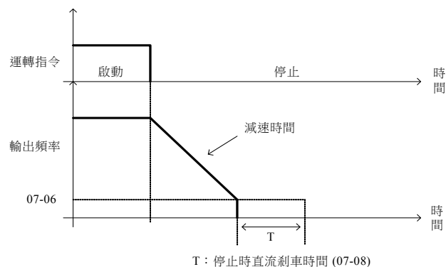
圖 4.3.58 減速停止
